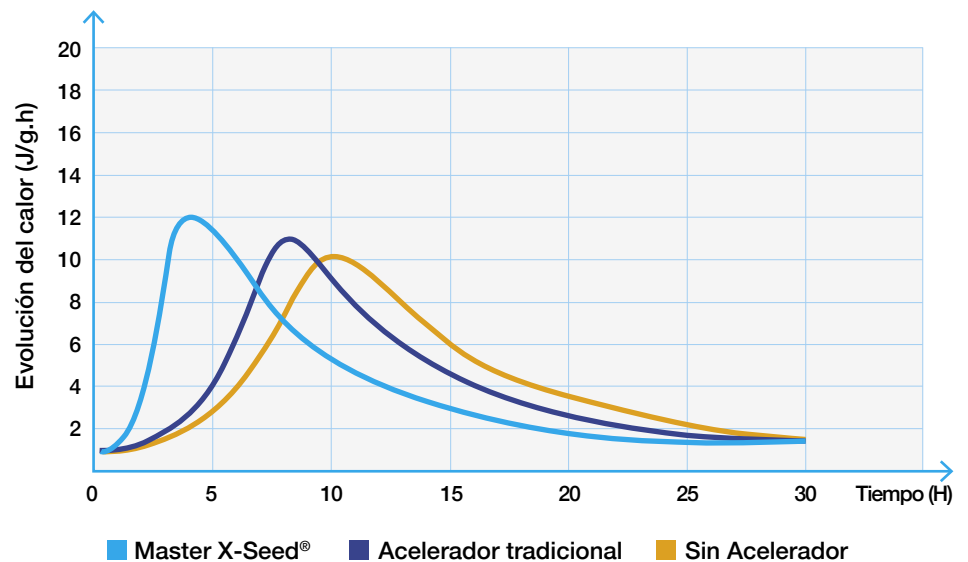
Evolución de temperatura – Efecto de acelerante (380 kg/m 3 CEM I 52.5R)
