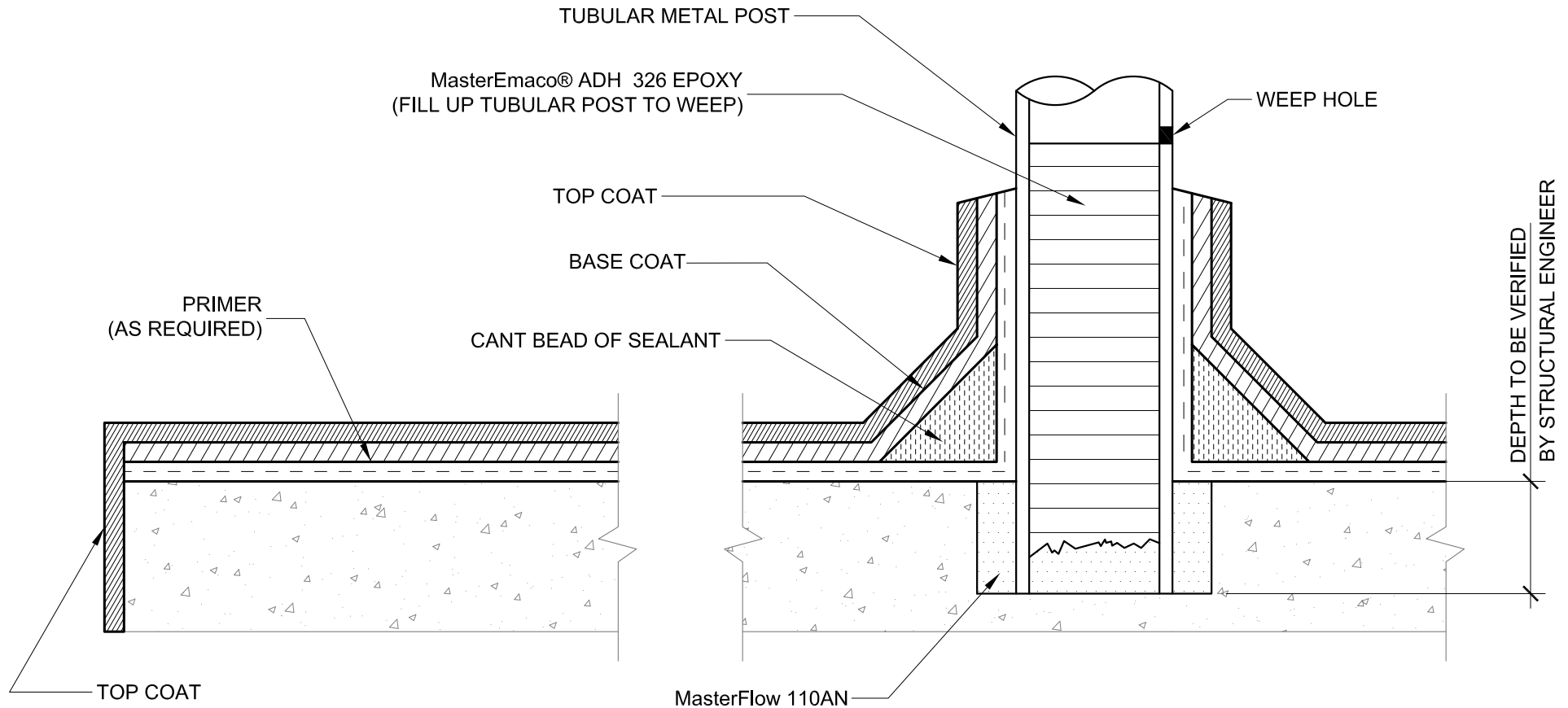
BALCONY EDGE - DC-13 N.T.S.
